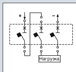
750 В пост. тока (3P)
