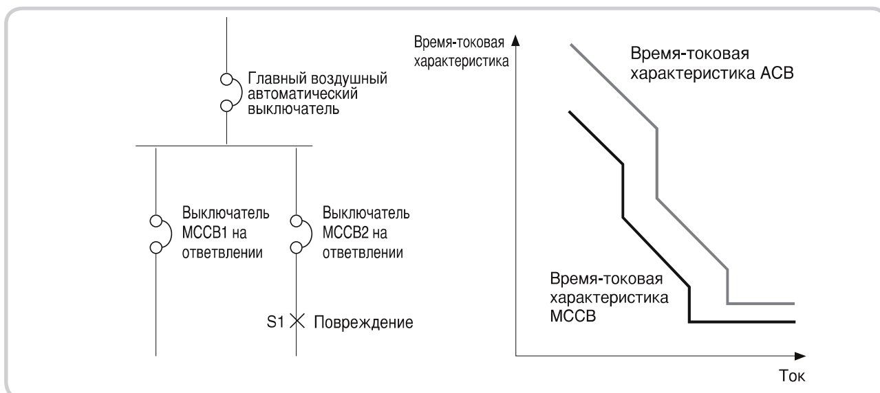
Рис. 2. Селективная защита
