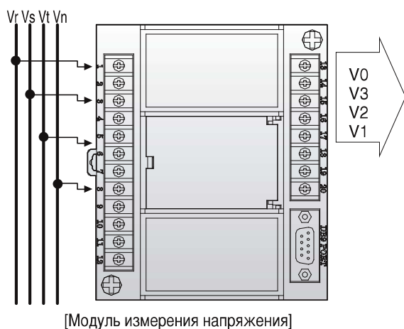
3-фазная 4-проводная сеть
