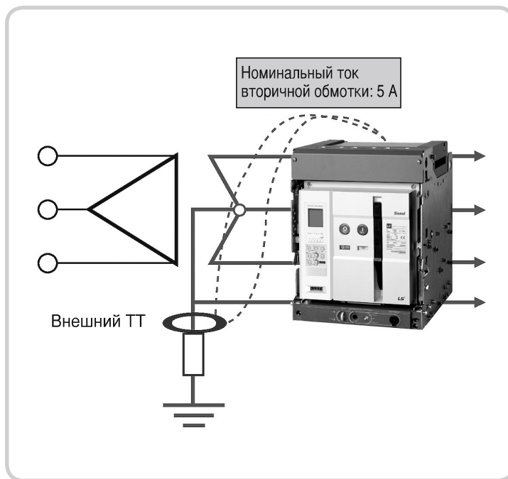
Внешний ТТ, схема 2
