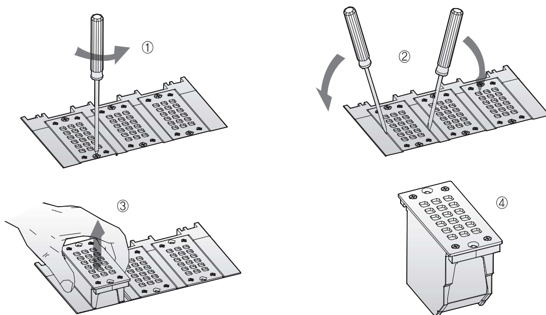
Рис. 7. Демонтаж дугогасительной камеры
