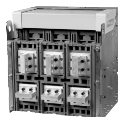
Рис. 3 Горизонтальные и вертикальные выводы для заднего присоединения шин
