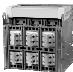
Рис. 2 Вертикальные выводы для заднего присоединения шин
