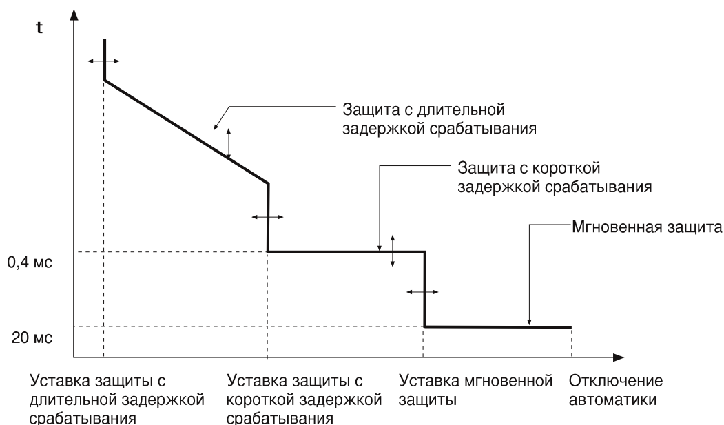
Рисунок 1. Время-токовая характеристика автоматического выключателя низкого напряжения
