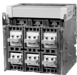
Рис. 1 Горизонтальные выводы для заднего присоединения шин
