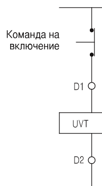
Принципиальная схема
