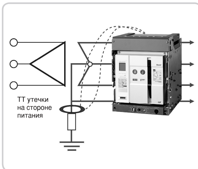
Схема 2
