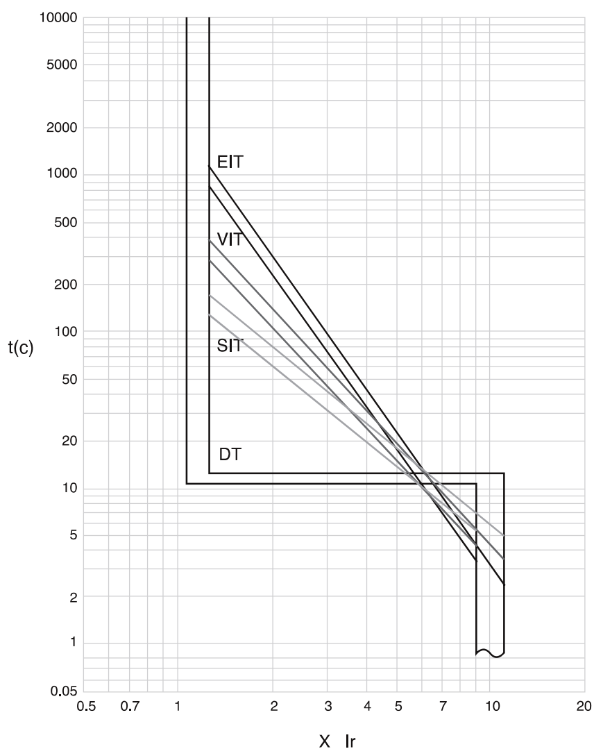
Рисунок 8. Характеристики IDMTL
