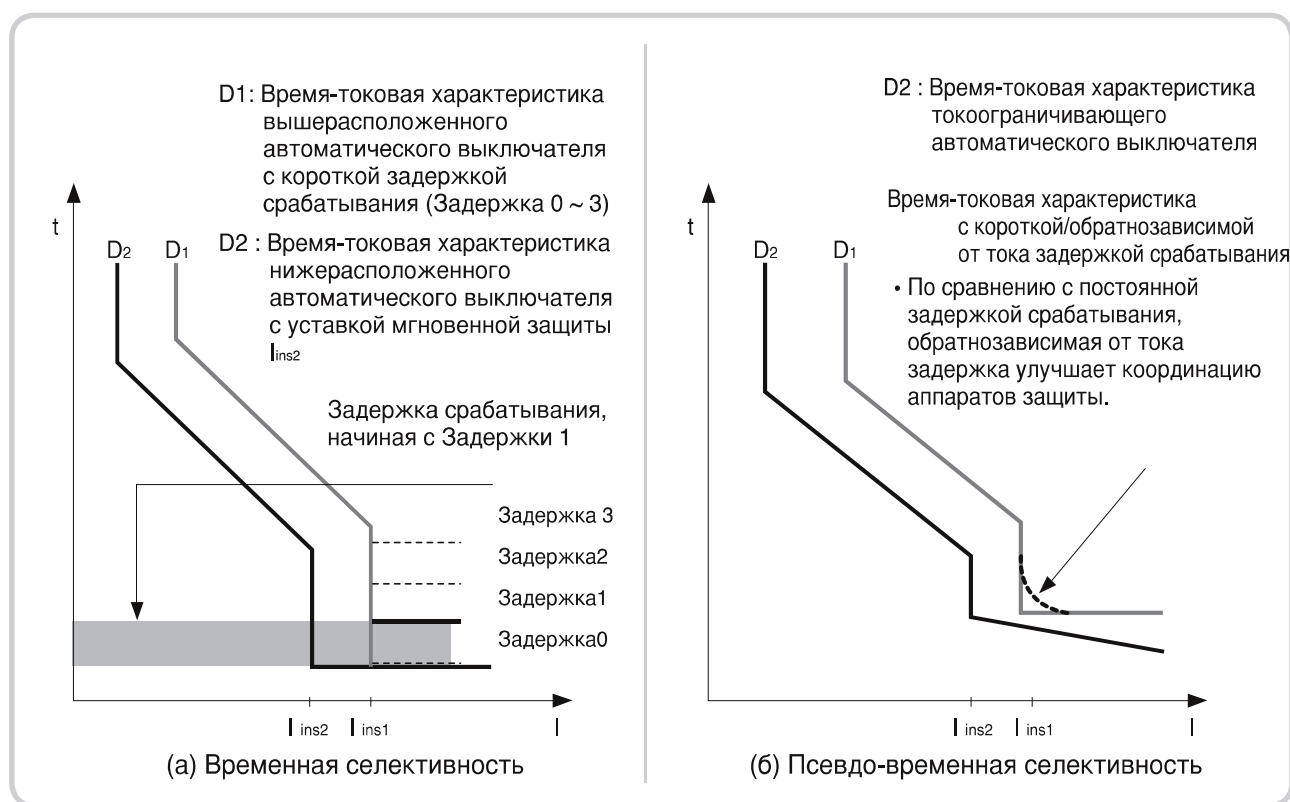
Рисунок 4. Временная селективность
