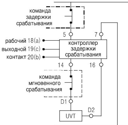
Принципиальная схема
